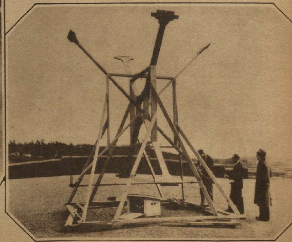
SE ESTA EXPERIMENTANDO este curioso aparato en varios aerodromos de Estados Unidos, para orientar a los pilotos y ayudarles a aterrizar en la niebla.
